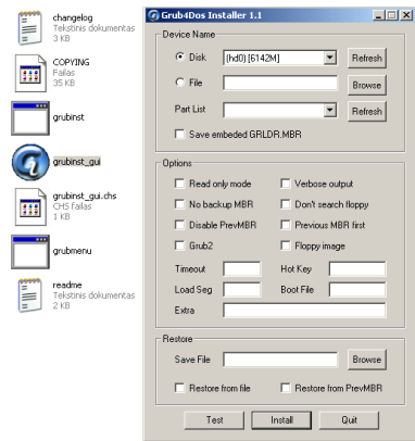
2. pav.: grubinst_gui programa
